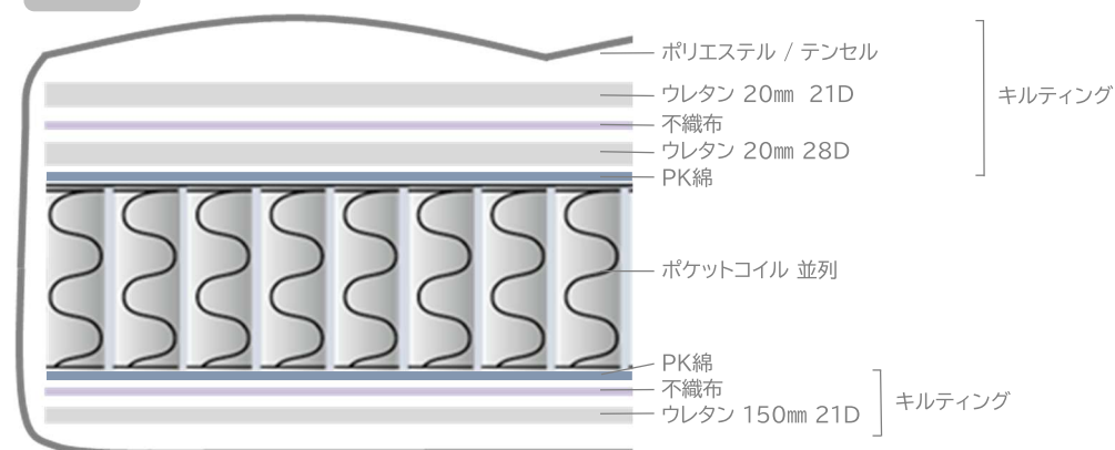
断面図
